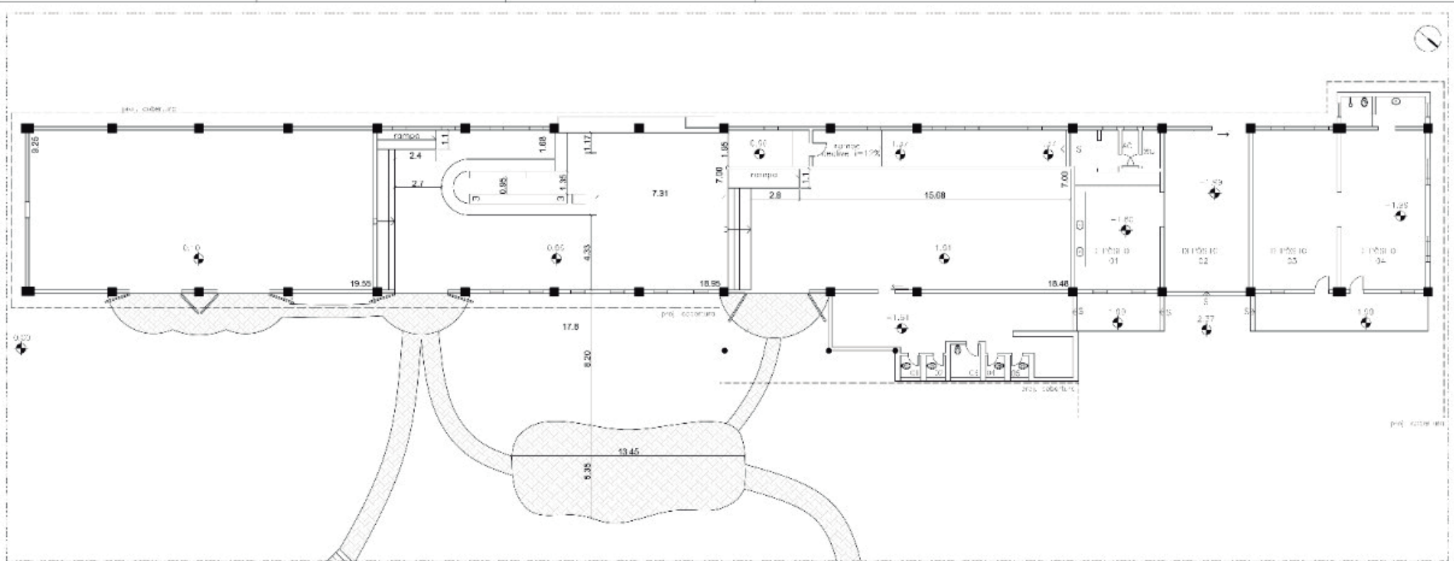
0 2 5 10 PLANTA CELEIRO E JARDIM EXTERNO ESC 1:150
