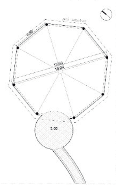
0 2 5 10 PLANTA GAZEBO ESC 1:150
